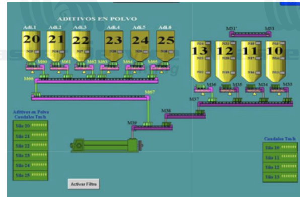
Implementación de la lógica de control
