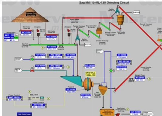
Diseño de sistemas SCADA
